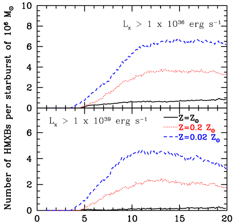
Linden et al. 2010
