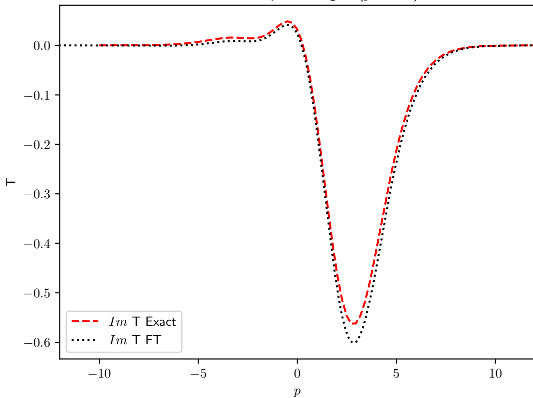
Im T exact vs path integral ( p = 1.0 )
