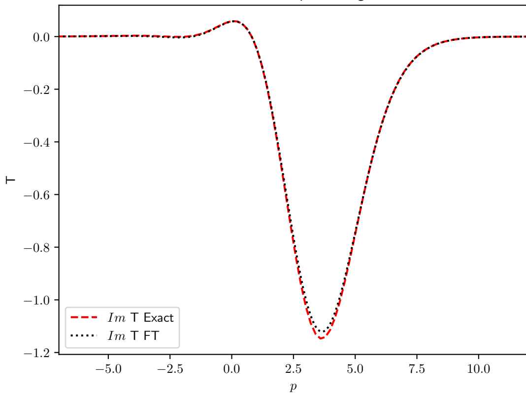
Im T exact vs path integral
